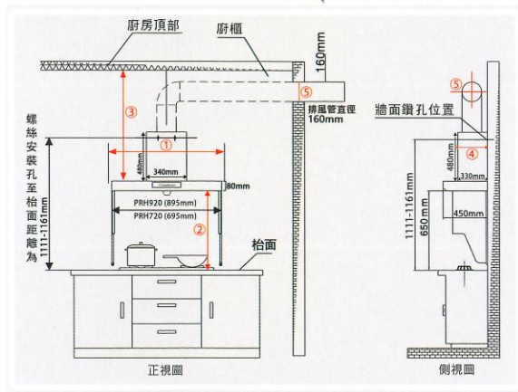
PRH720A/PRH920 安裝示意圖
