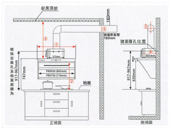
PRH730/PRH930 安裝示意圖
